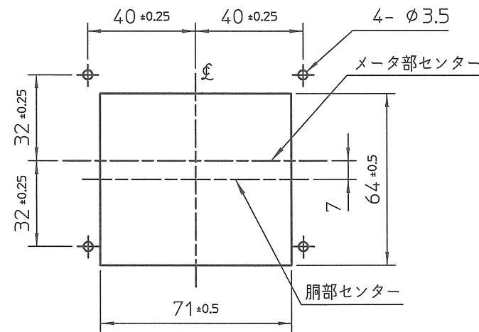
パネルカット寸法
