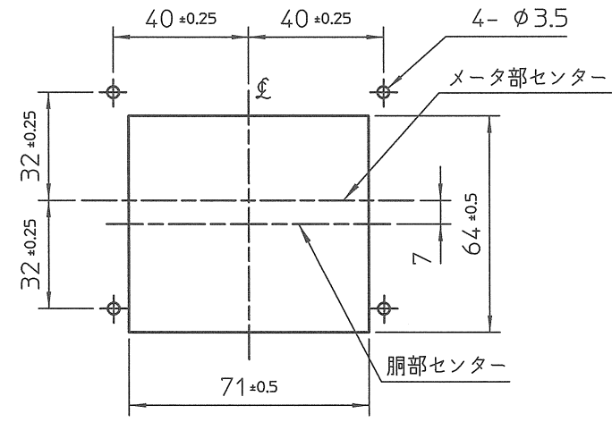
パネルカット寸法
