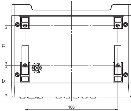
Screw hole position for Rack-mounted ラックマウント用底面ネジ穴位置
